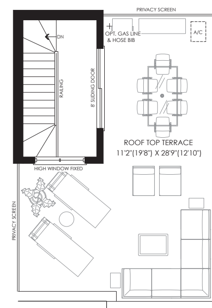
ROOF TOP TERRACE ELEV. 'A','B'
